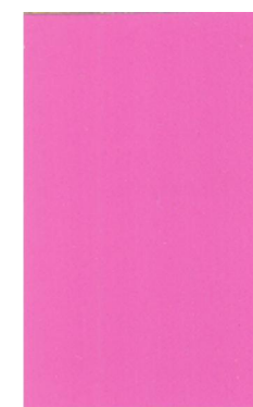
Reduction (1:16 TiO 2 )
